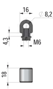
Rod Adapter
